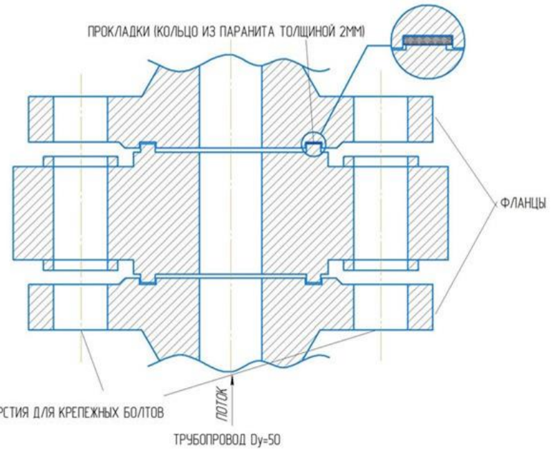
СХЕМА МОНТАЖА ПЕРВИЧНОГО ПРЕОБРАЗОВАТЕЛЯ
