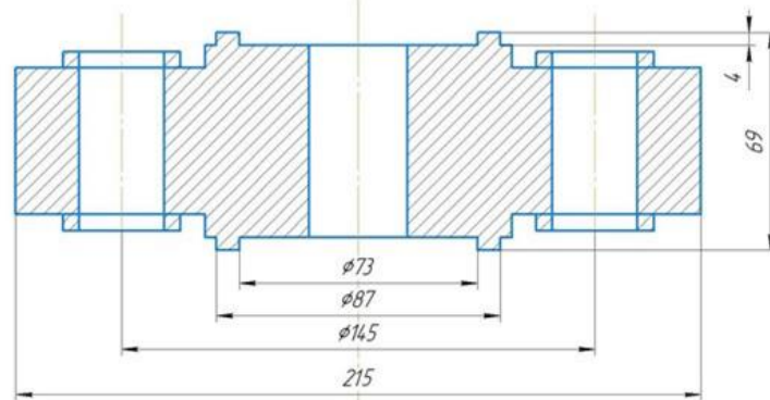
ПЕРВИЧНЫЙ ПРЕОБРАЗОВАТЕЛЬ
