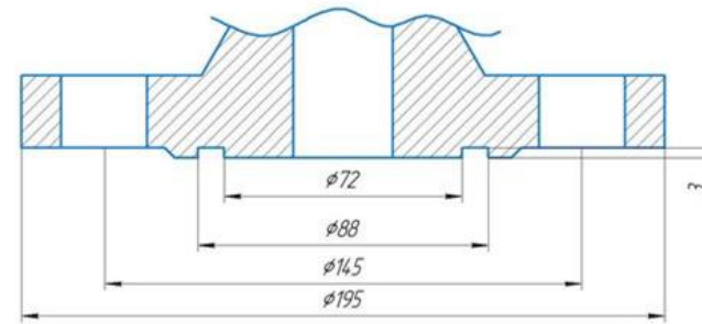
ПРОКЛАДКИ (КОЛЬЦО ИЗ ПАРАНИТА ТОЛЩИНОЙ 2ММ)
